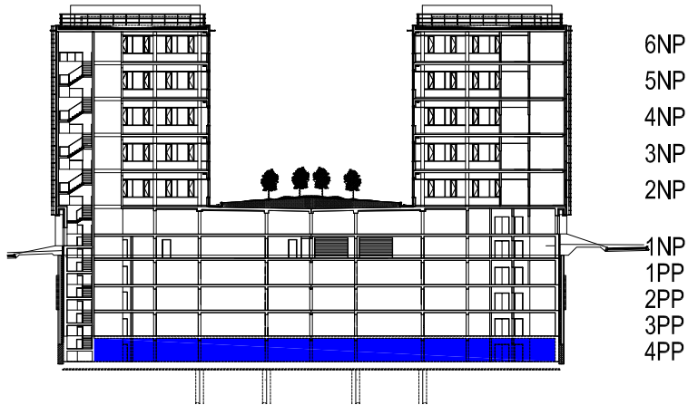
UMÍSTĚNÍ V POSCHODI
